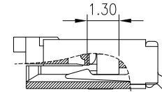
CABLE INSERT DIM.
